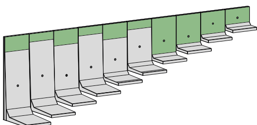
Elementen van verschillende hoogte op een getrapte fundering
