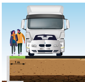
LVF-ASSORTIMENT zwaar verkeer, gelijkmatig verdeelde bovenbelasting volgens NEN EN 1991-2
