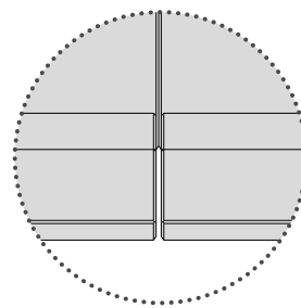
Onderaan de voet is een zandspleet gemaakt om de wanden gemakkelijker te plaatsen zodat de bovenzijden mooi aansluiten.
