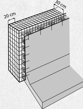
DÉPASSANT LATÉRAL: Colonne + fixation avec plaquette en galva et vis
